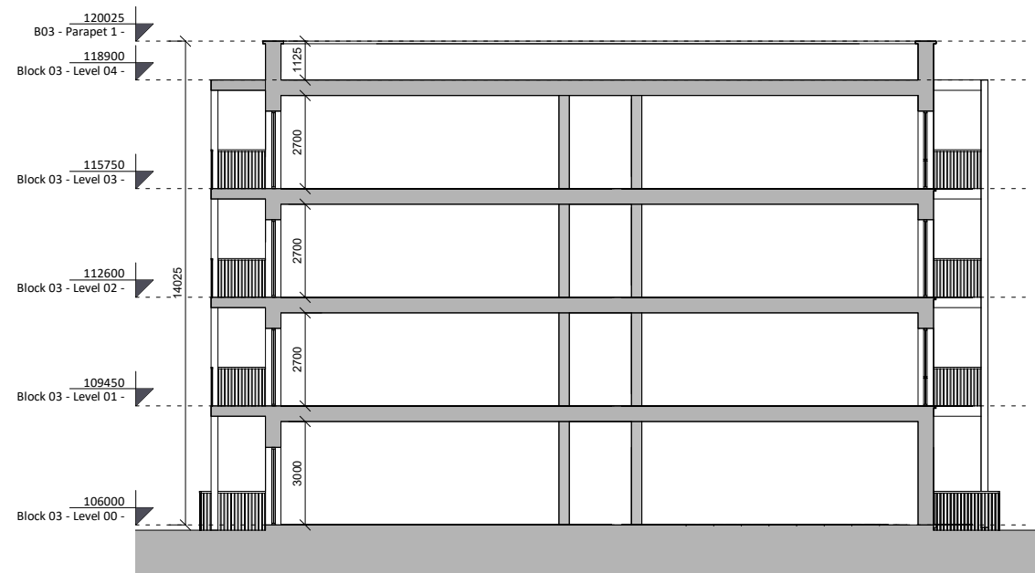
③ Block 03 - Section A-A 1 : 200
